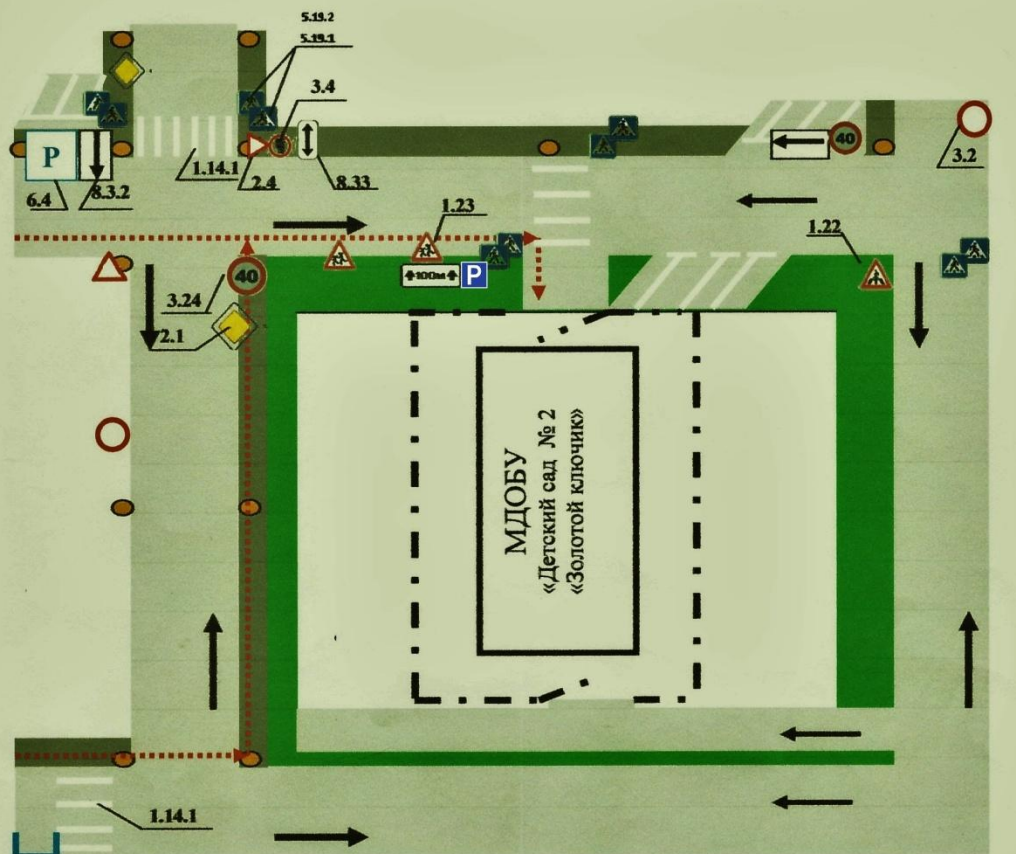
2. Схема организации дорожного движения в непосредственной близости от образовательного учреждения с размещением соответствующих технических средств организации дорожного движения, маршрутов движения детей и расположения парковочных мест
